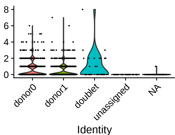
DQA1.02.01.23
