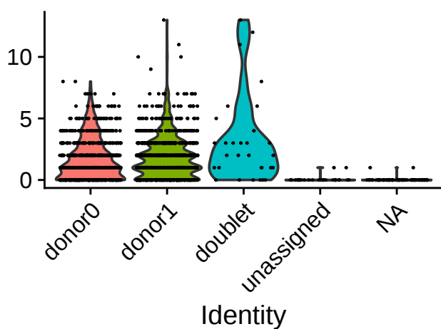
B.08.78
