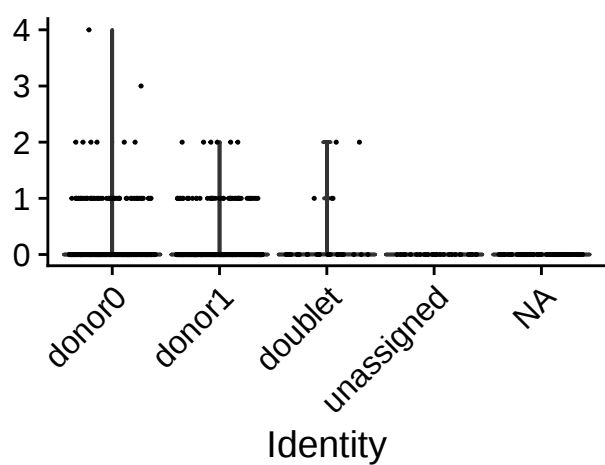
DPA1
