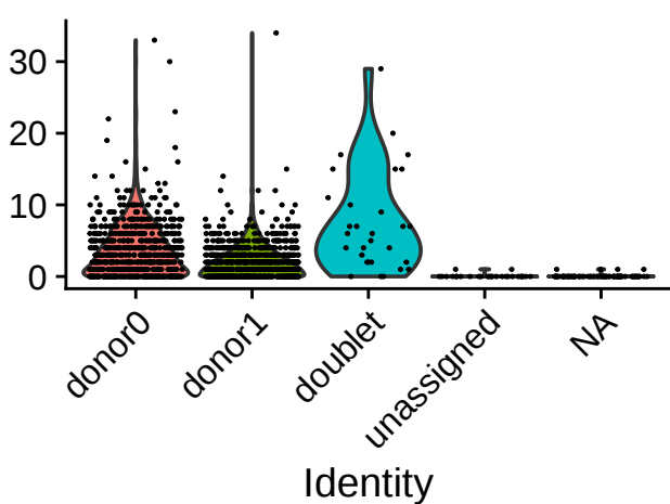
DRB1.03.01.38
