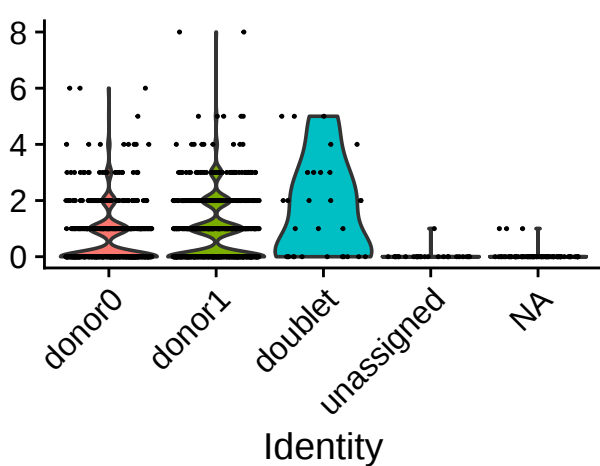
DQB1.02.01.40
