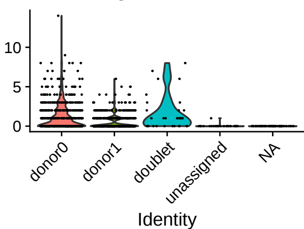
DRB1.03.01.38
