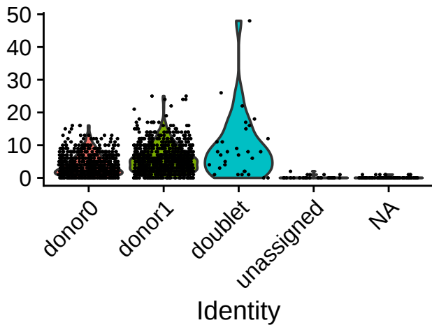
DPA1.02.49
