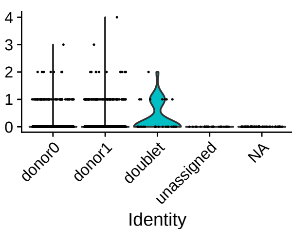
C.04.01.88
