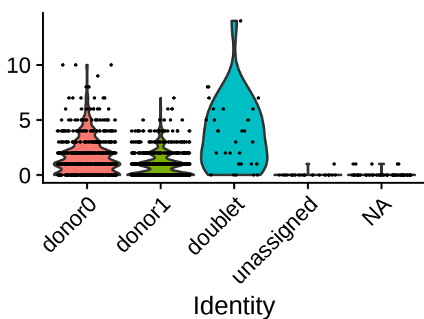
DQB1.02.01.40
