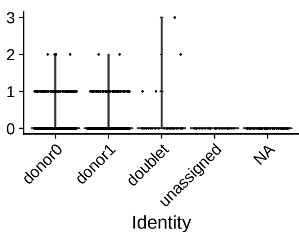
DPA1.01.107.01.01
