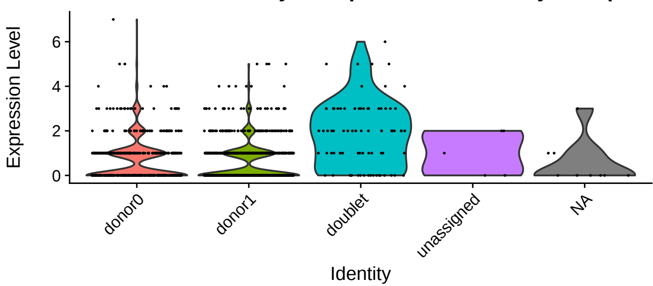
B-07:02:01:01-PASC-Sample-D
