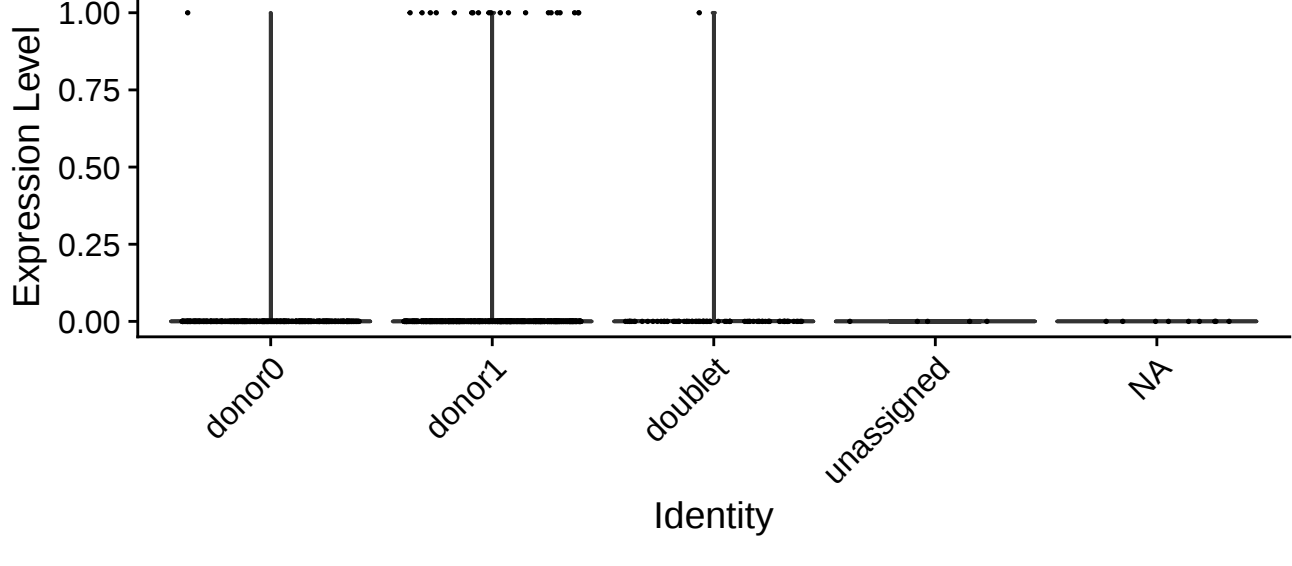
A24:02:01:04-PASC-Sample-D
